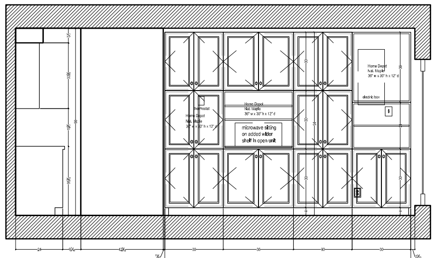
6 ELEVATION
