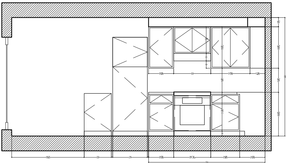
3 ELEVATION
