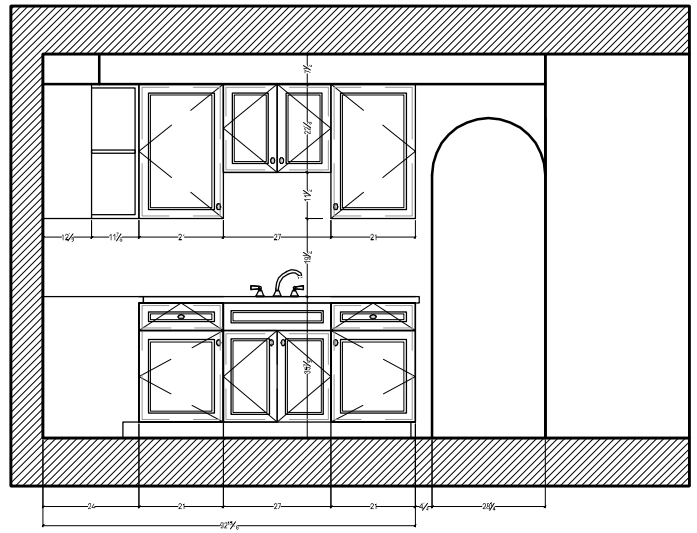
2 ELEVATION
