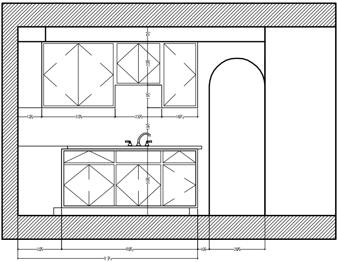
1 ELEVATION
